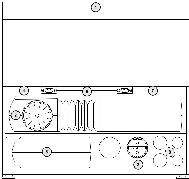
Universaltragtasche F2000
